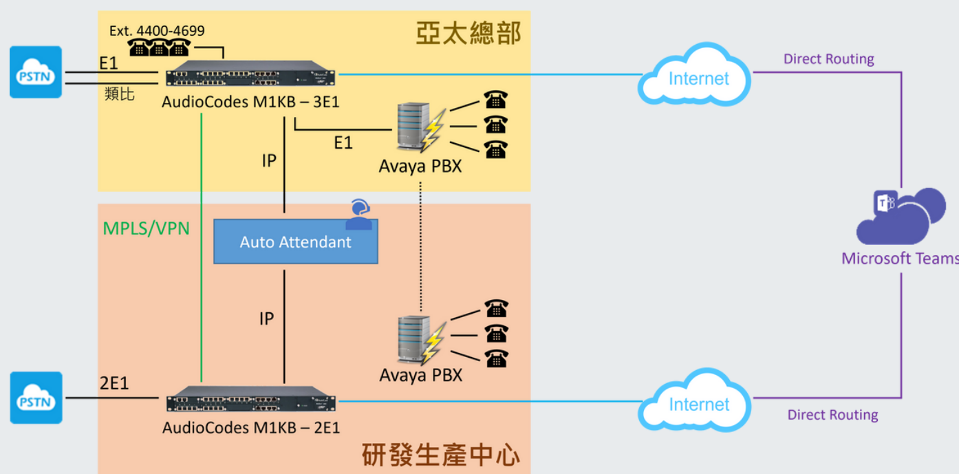
▲ 完成架構圖
